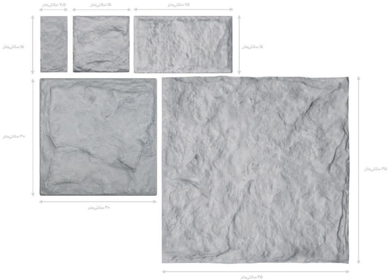
دیوارپوش بادبر ۱۵×۷٫۵ - ۱۵×۱۵ - ۲۵×۱۵ - ۳۰×۳۰ - ۴۵×۴۵
